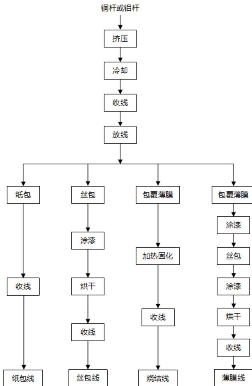
图 3-3 绕包线生产工艺流程图
