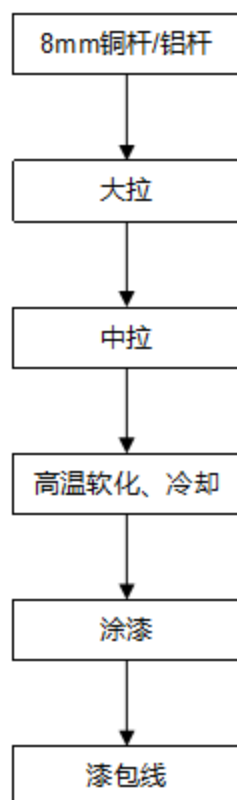
图 3-2 漆包线生产工艺流程图
