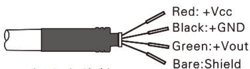
电压型3线制
