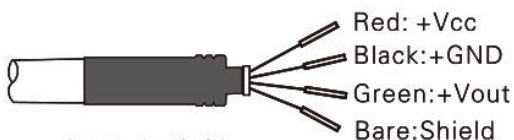
电压型3线制
