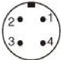
M12连接器
