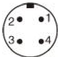
M12连接器
