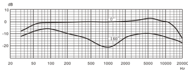
话筒杆频响特性:
