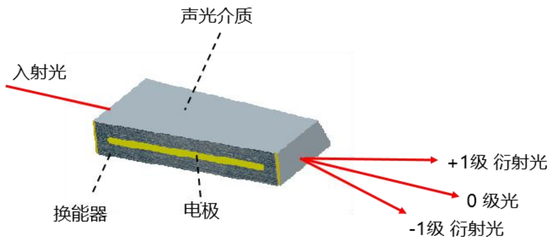
声光Q开关示意图
