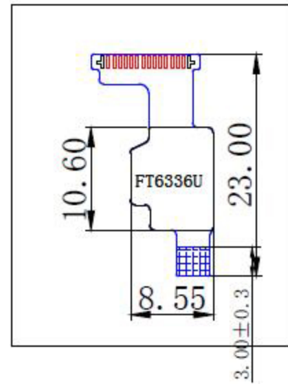
FPC 背视图1:1
