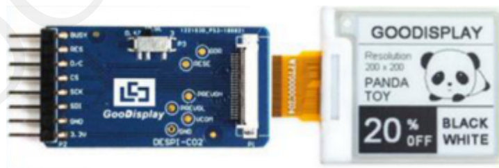
图4 电子纸与转接板插接示意图
