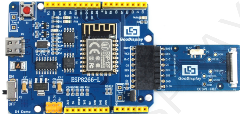
图 3 主板与转接板连接方式
