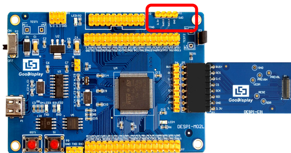
图 10 SWD 接口
