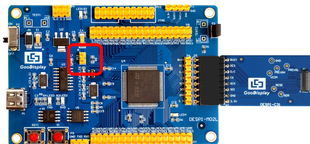
图 11 P12 短接位置
