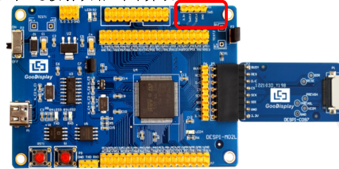
图 10 SWD 接口
