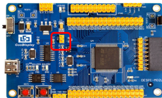
图 11 P12 短接位置
