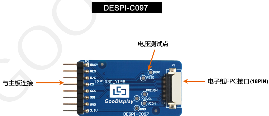
图 2 转接板 DESPI-C097功能图
