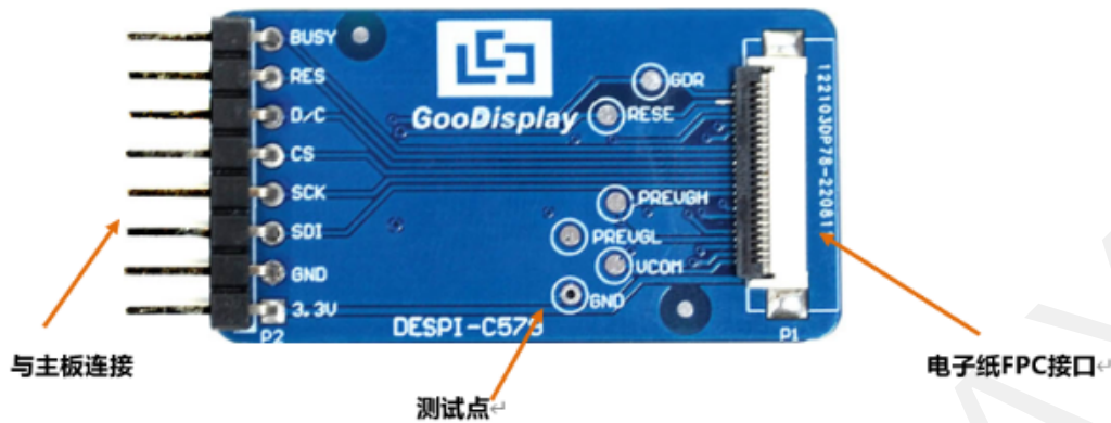
图 1 主转接板 DESPI-C579 功能图
