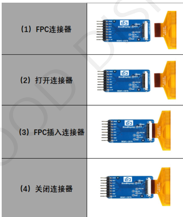
图 2 电子纸显示屏与转接板连接方式
