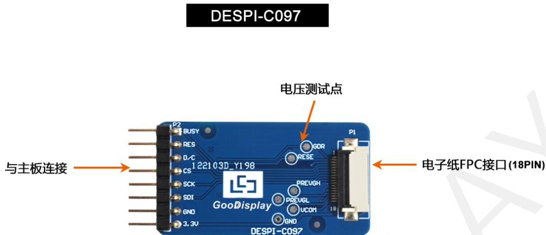
图 1 转接板 DESPI-C097(18PIN)功能图
