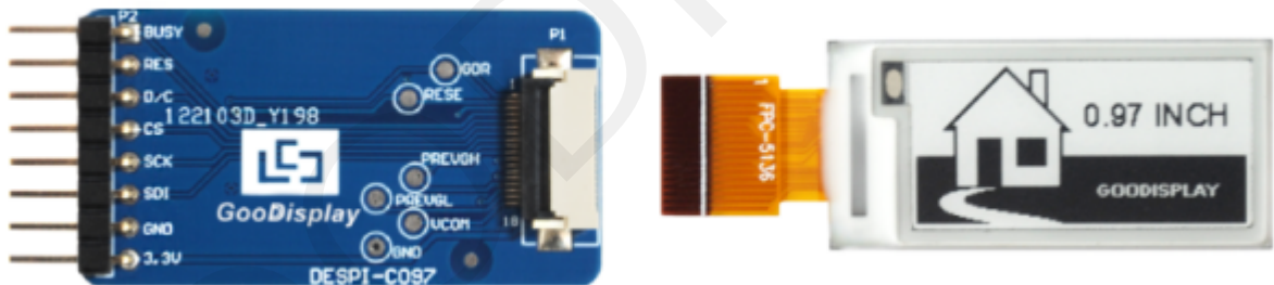
图 2 电子纸显示屏与转接板连接方式
