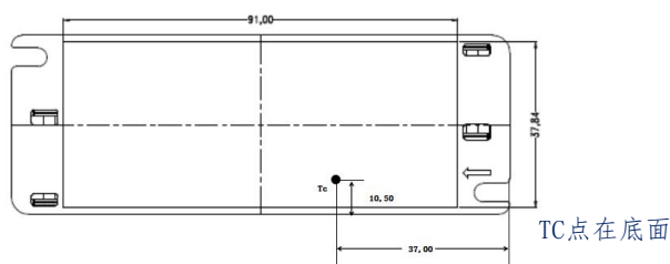
底视图
