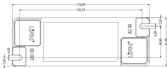
俯视图
