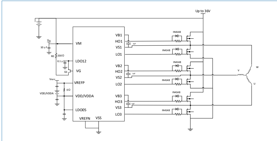
图 5-2 典型应用框图
