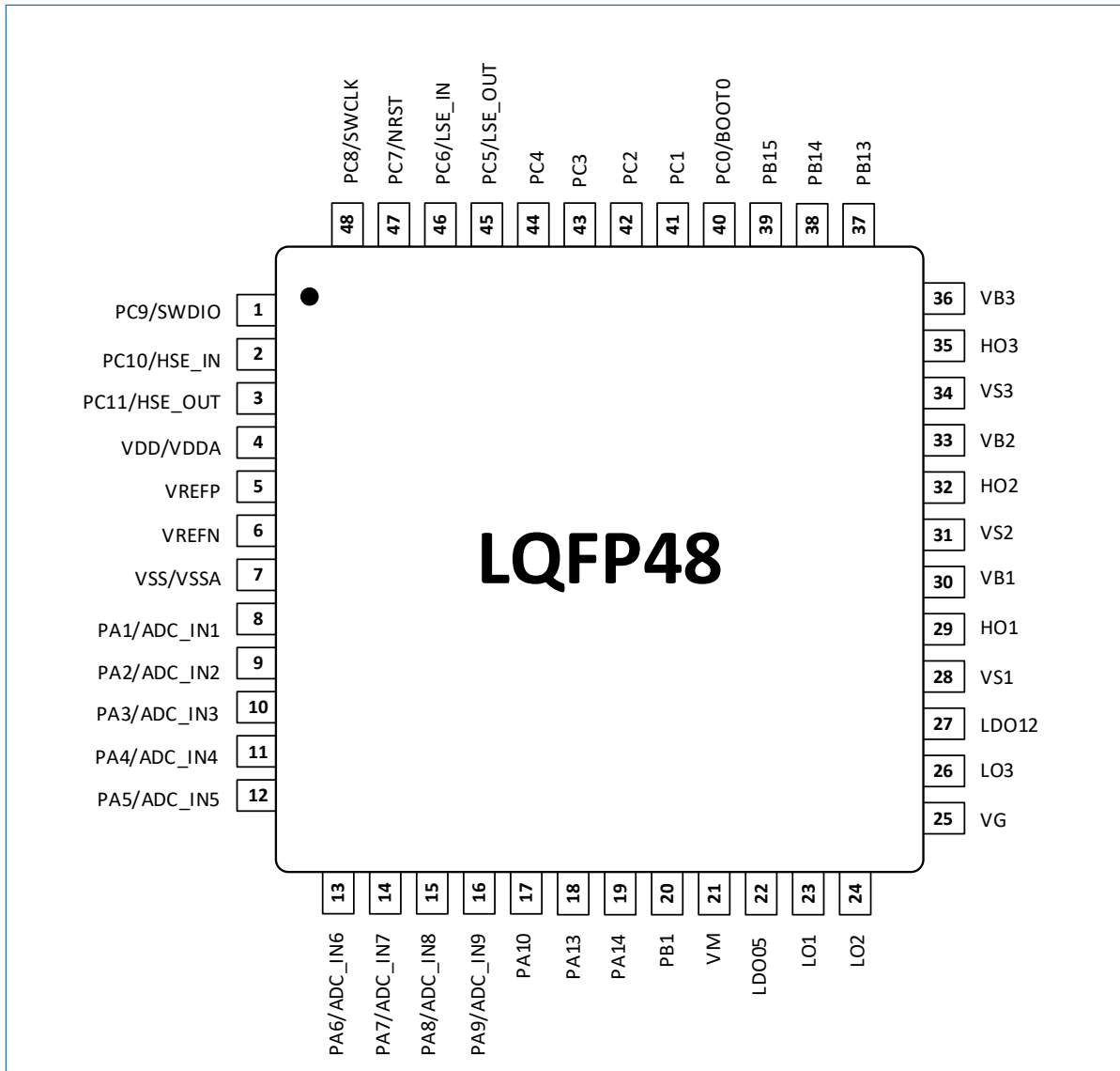
图 6-1 LQFP48 封装引脚排列
