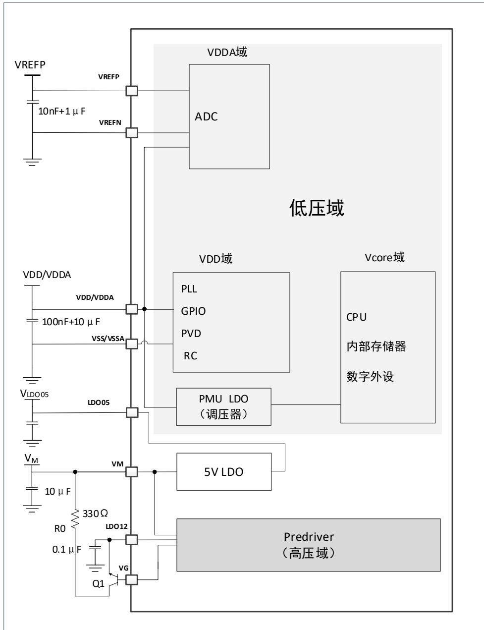
图 5-1 电源框图
