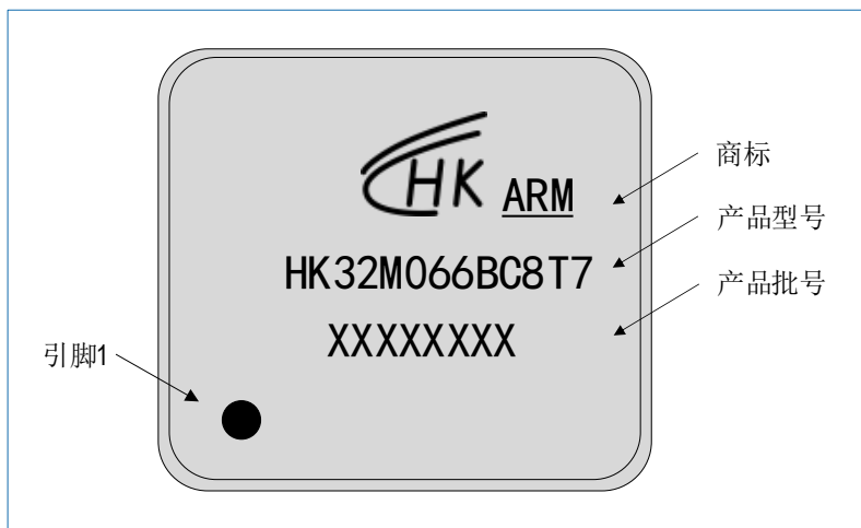
图 7-2 LQFP48 HK32M066BC8T7 丝印示例
