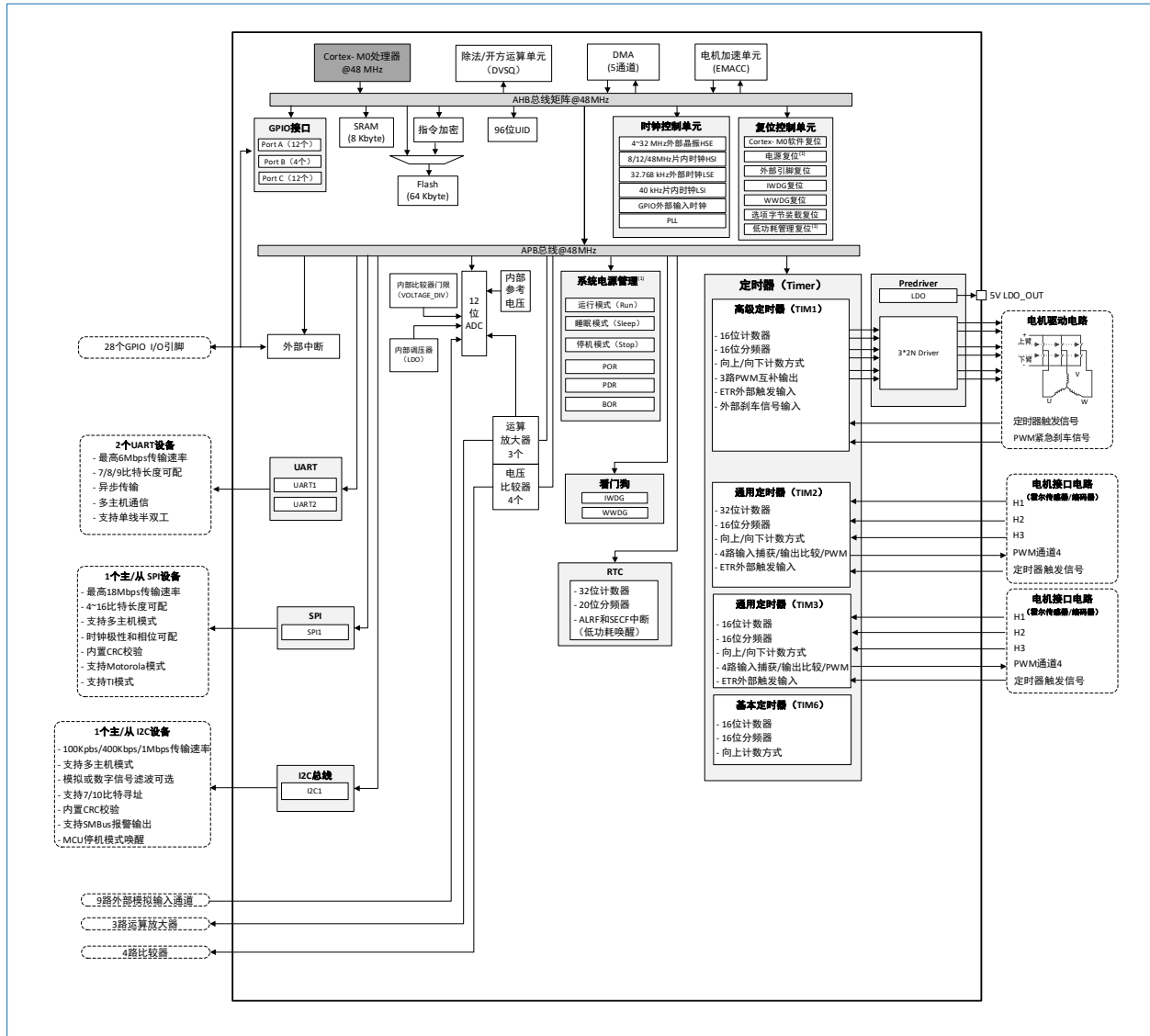
图 3-1 HK32M066B 功能框图
