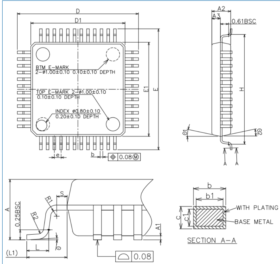
图 7-1 LQFP48 封装尺寸
