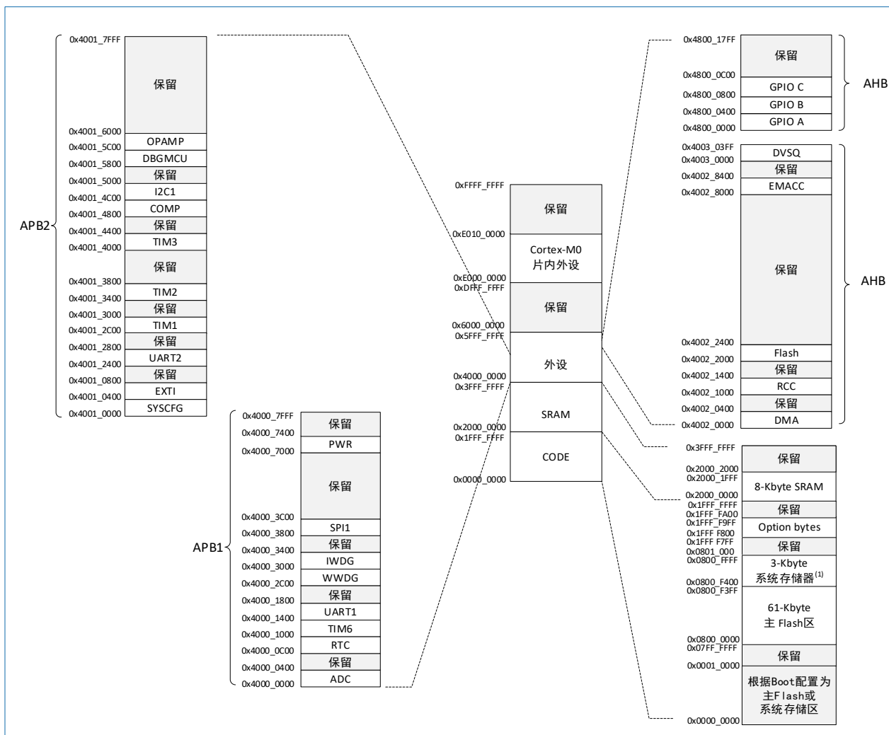
图 3-2 HK32M066B 存储器映射
