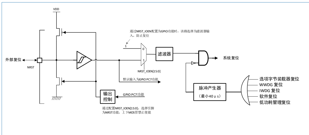
图 3-3 复位信号
