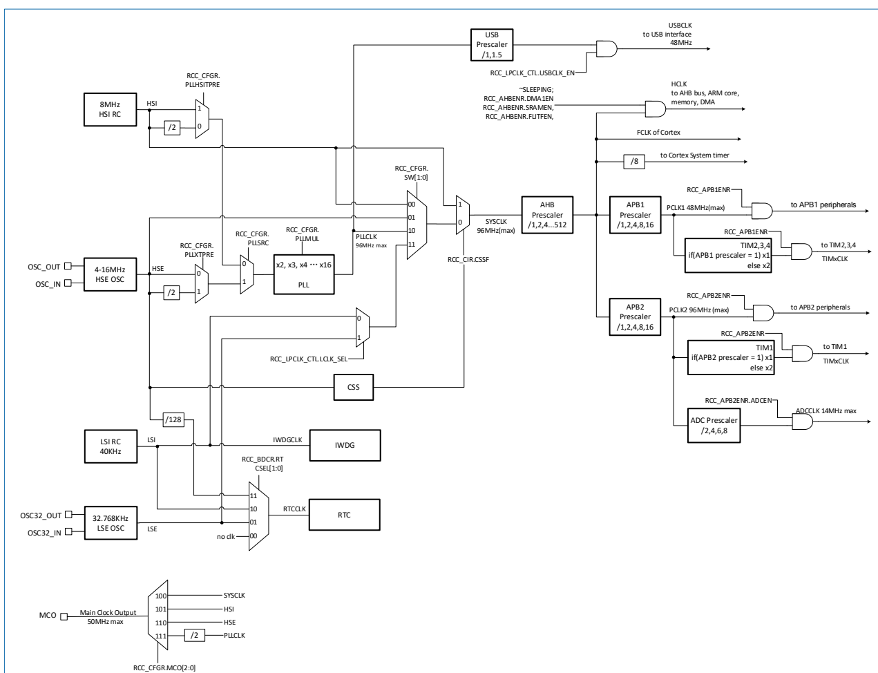
图 3-4 时钟树
