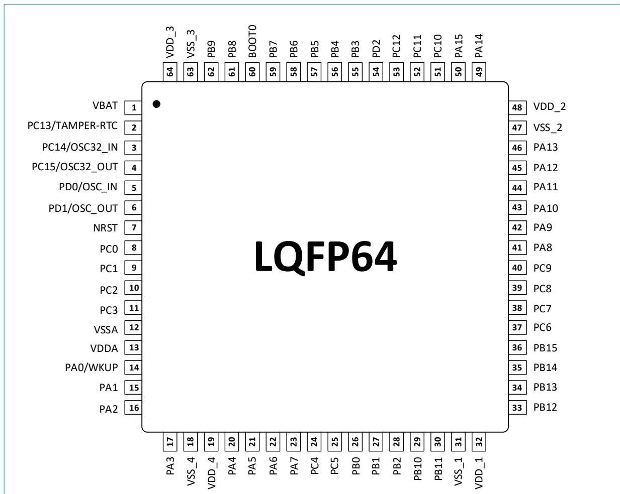
图 5-1 LQFP64 封装
