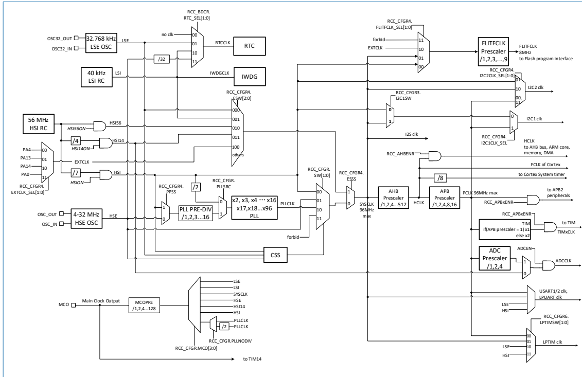
图 3-4 HK32F072x8xB 时钟树
