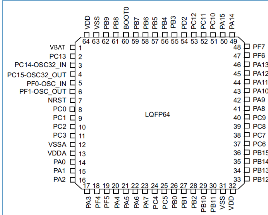
图 6-1 LQFP64 (HK32F072RxT6) 封装管脚排列
