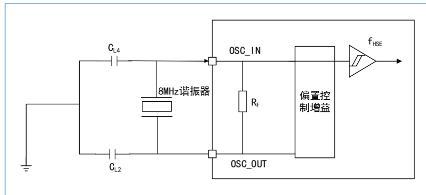
图 4-1 HSE 负反馈晶体振荡电路
