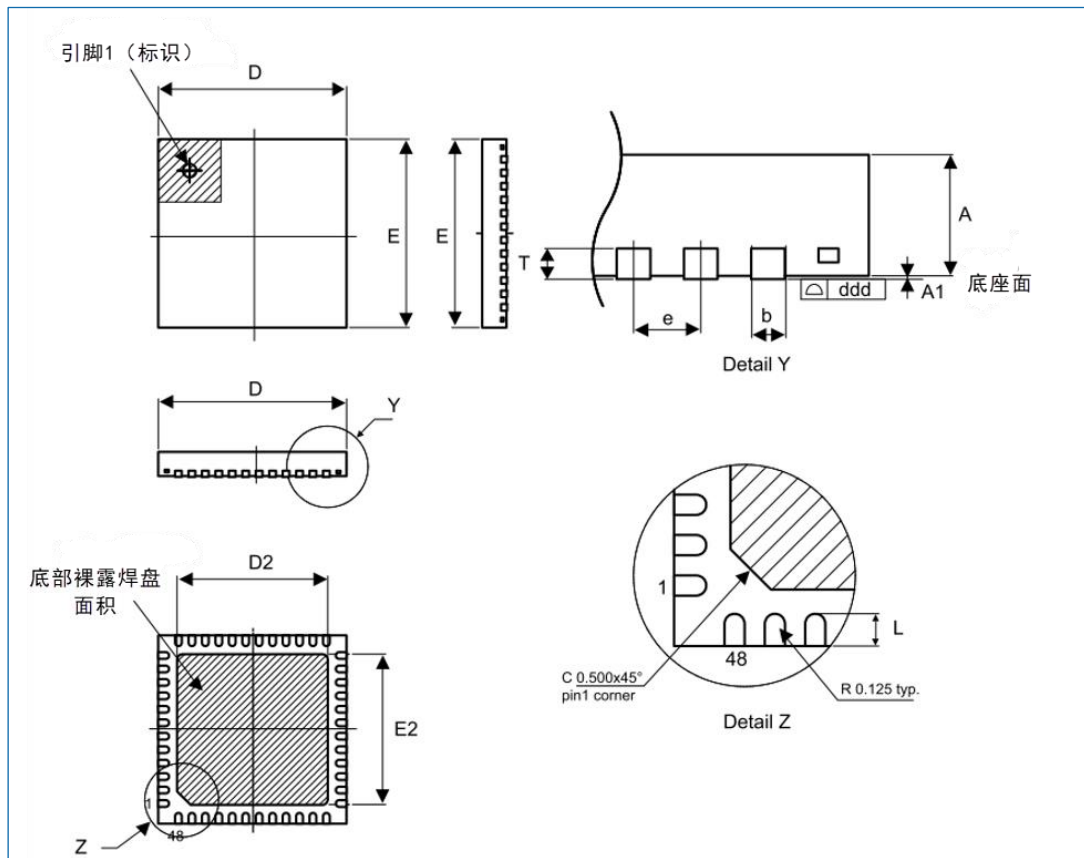
图 7-3 LQFP48 封装尺寸
