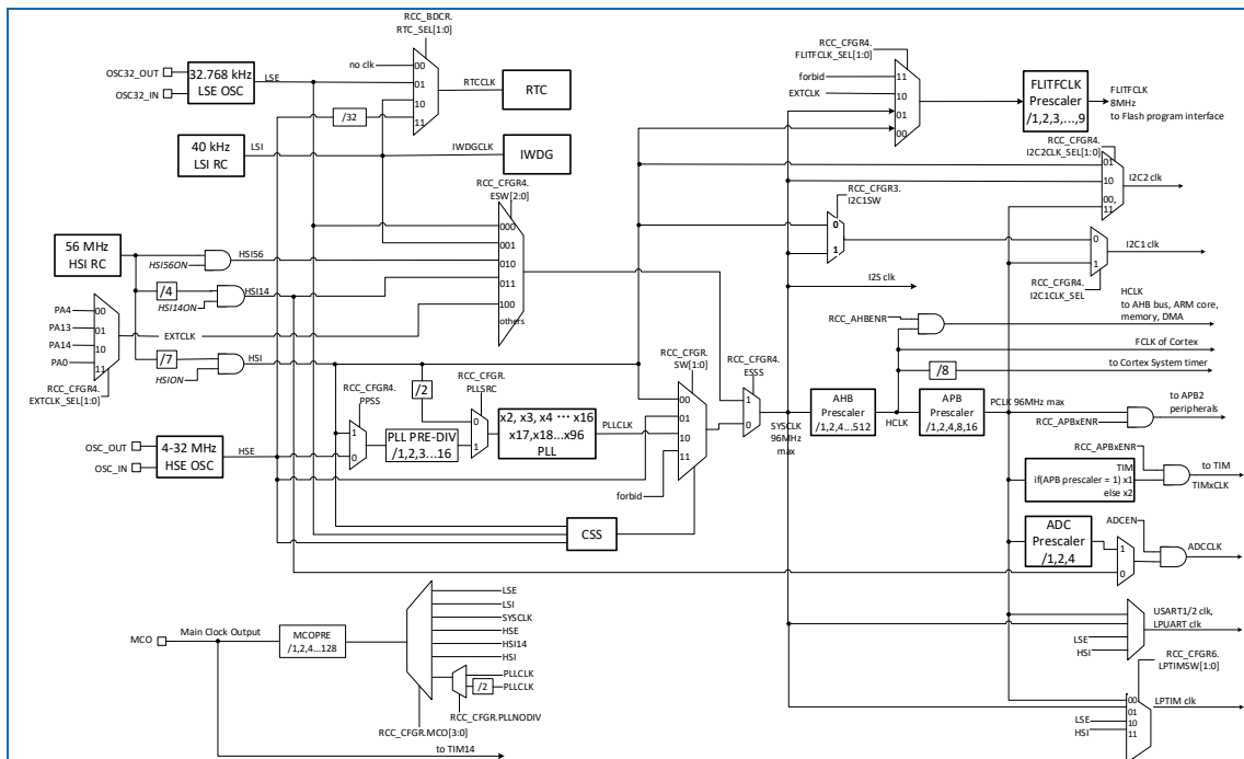
图 3-4 HK32F072x8xB 时钟树
