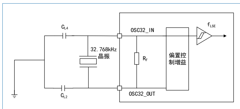
图 4-2 LSE 负反馈晶体振荡电路
