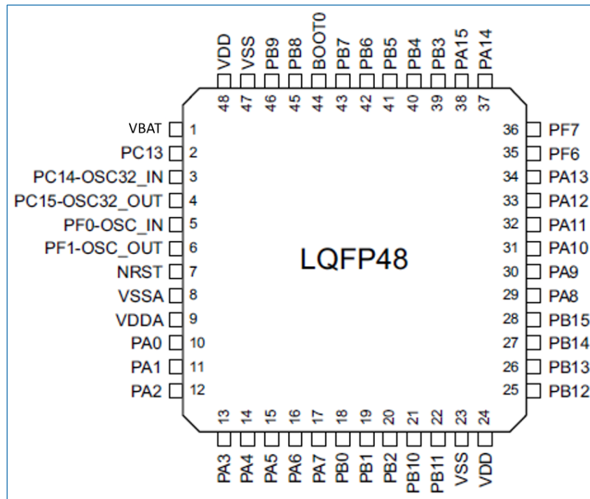
图 6-2 LQFP48 (HK32F072CxT6) 封装管脚排列
