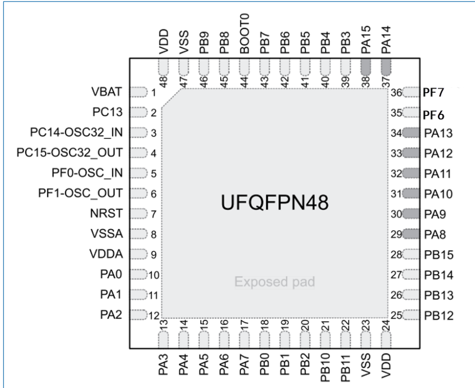
图 6-3 QFN48 (HK32F072CxU6) 封装管脚排列
