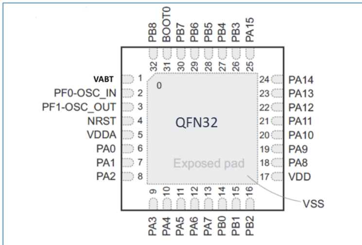
图 6-4 QFN32 (HK32F04AKxU6A) 封装管脚排列
