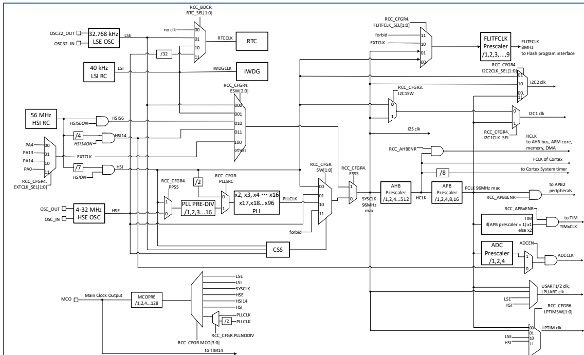
图 3-4 HK32F04AxxxxA 时钟树
