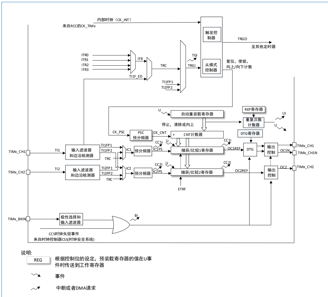
图 16-1 TIM15 框图
