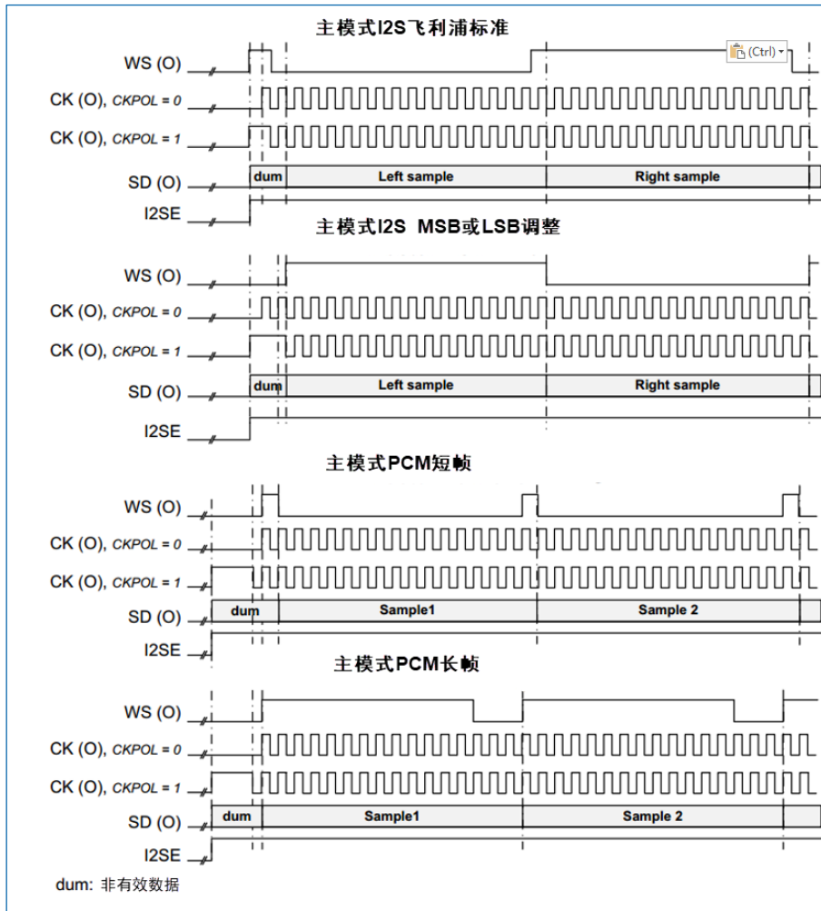
图 25-35 主模式下启动序列
