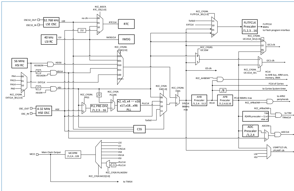
图 6-2 HK32F031xxxxA MCU 时钟树
