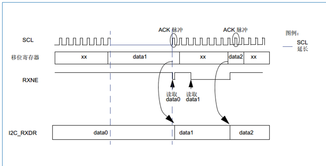
图 22-5 数据接收
