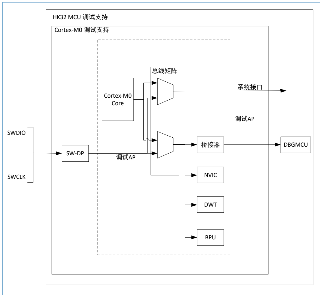
图 27-1 HK32F031xxxxA MCU 和 Cortex®-M0 级调试支持框图
