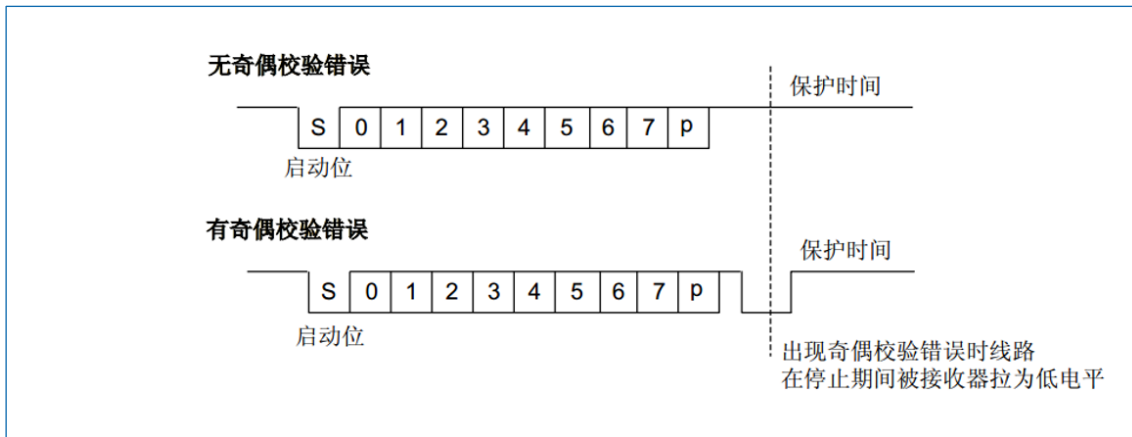
图 23-16 IS07816-3 异步协议
