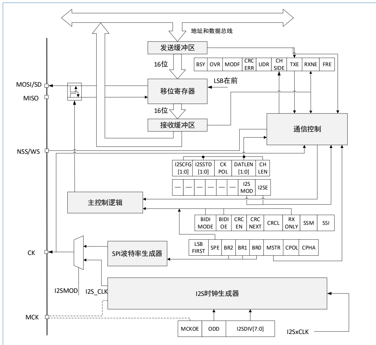
图 25-16 I2S 框图
