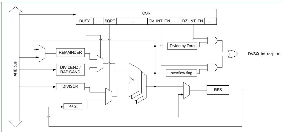
图 26-1 DVSQ 结构图
