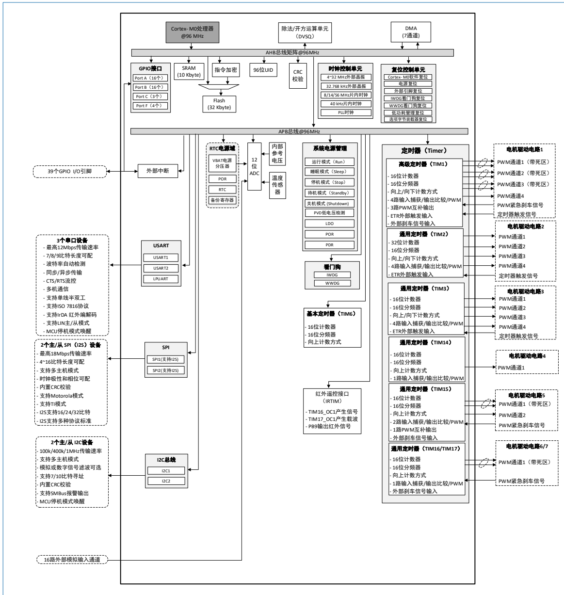
图 2-1 HK32F031C6T6A 功能框图
