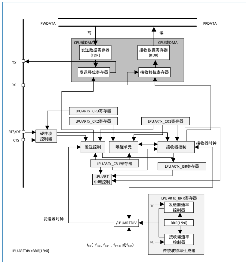
图 24-1 LPUART 框图
