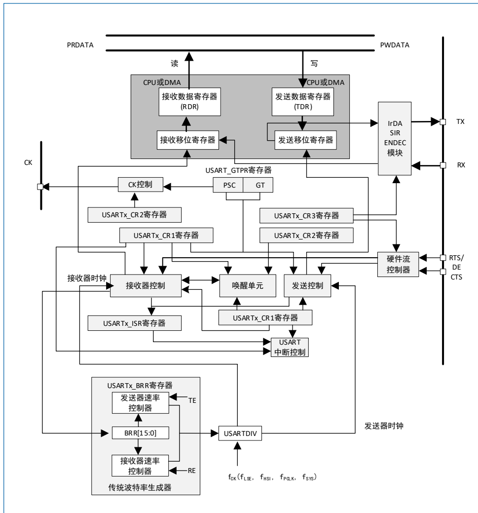
图 23-1 USART 框图
