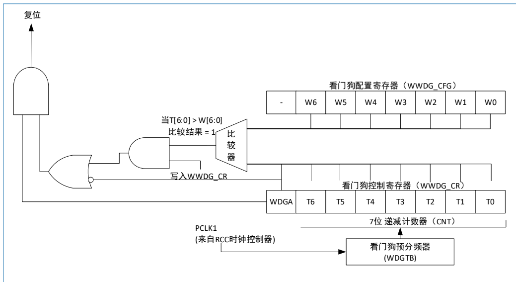
图 20-1 WWDG 框图
