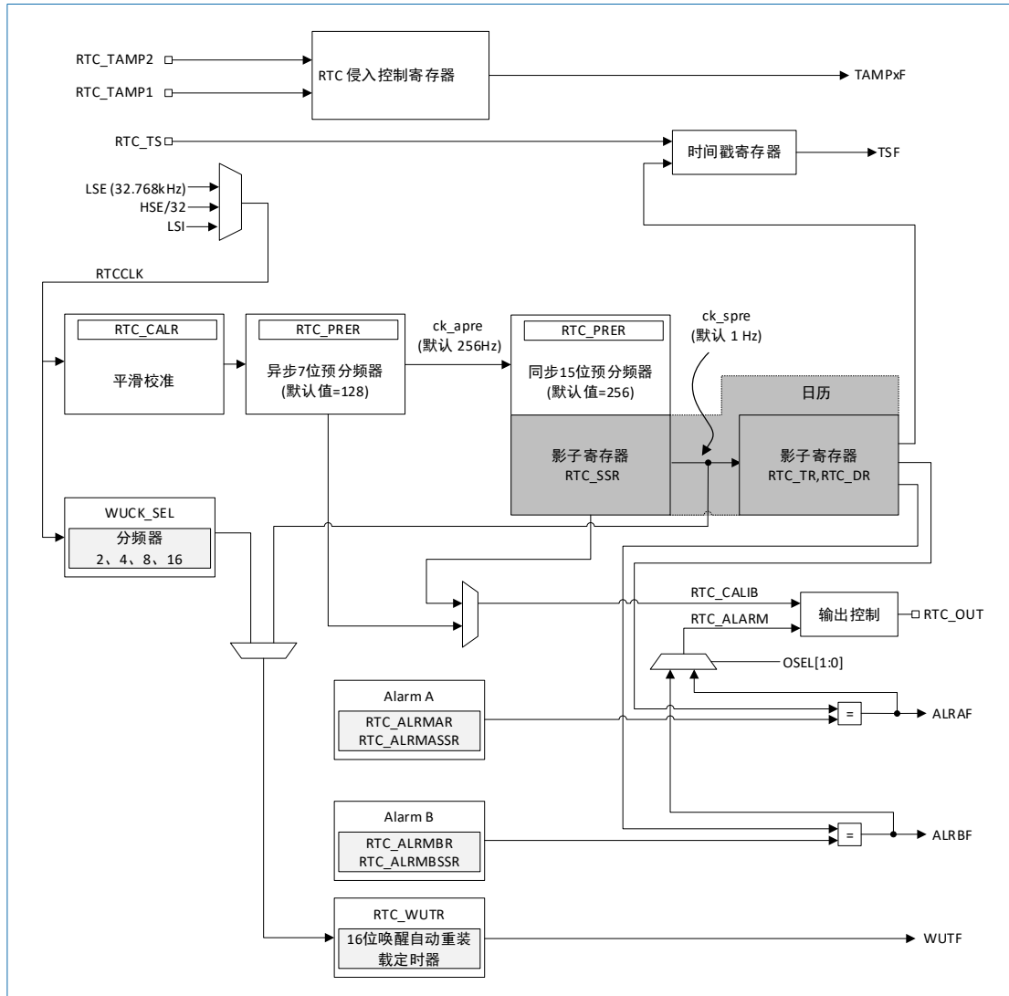
图 21-1 RTC 框图
