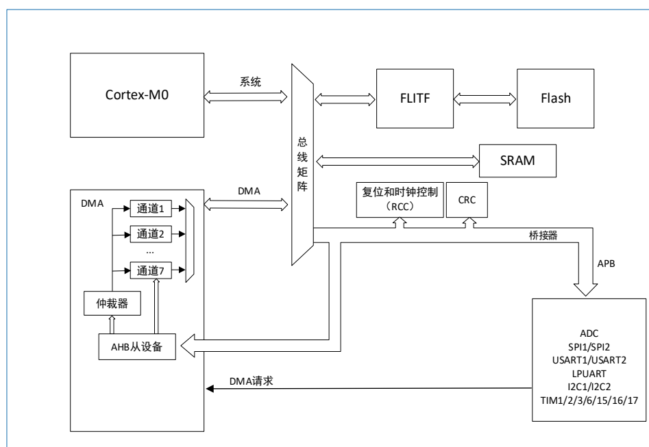
图 9-1 DMA 结构图
