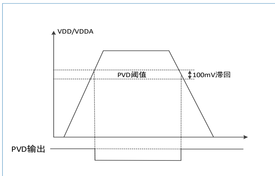
图 5-3 PVD 的门限
