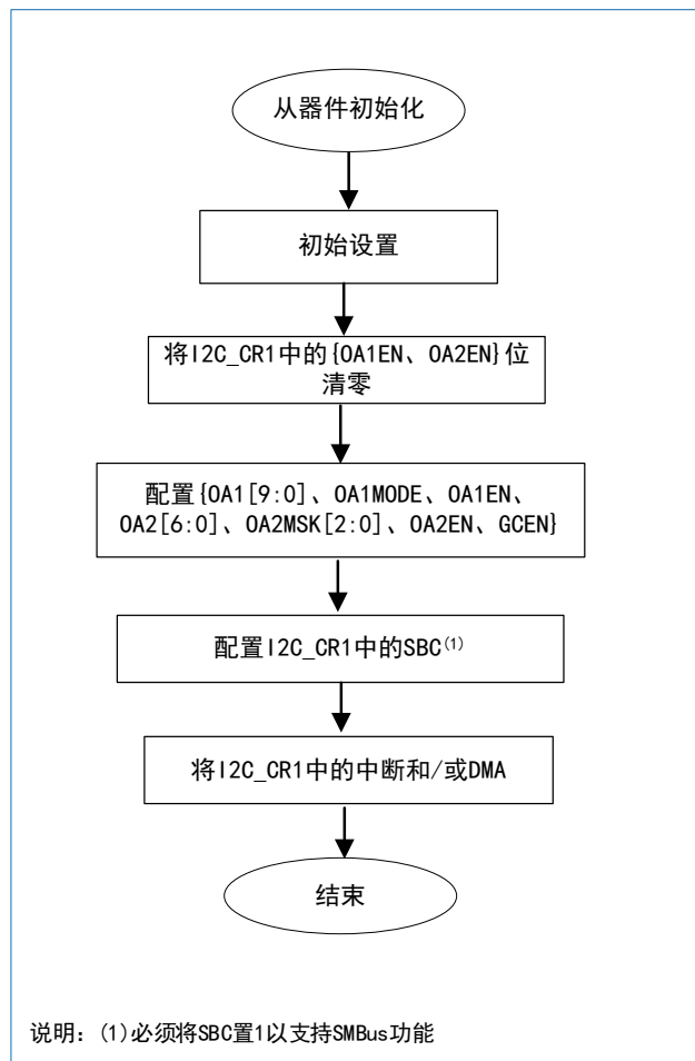
图 22-7 从器件初始化流程图
