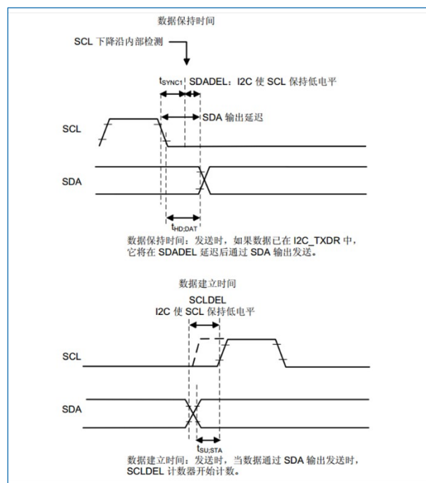
图 22-3 建立和保持时序
