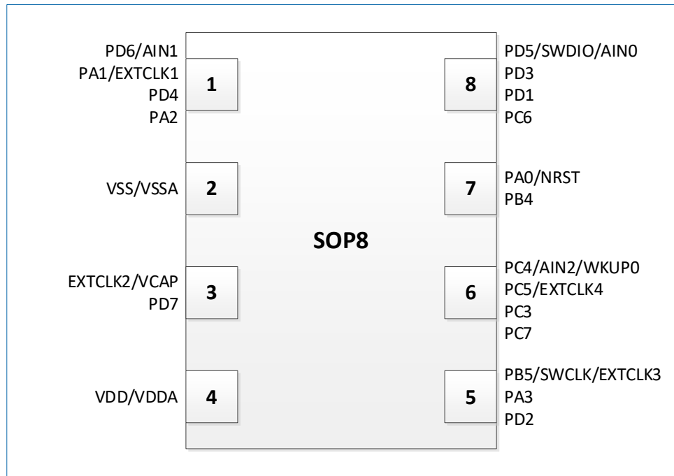
图 6-4 SOP8 封装
