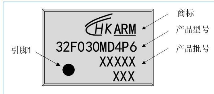
图 7-11 TSSOP16 HK32F030MD4P6 丝印示例
