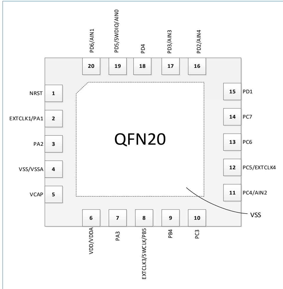
图 6-1 QFN20 封装
