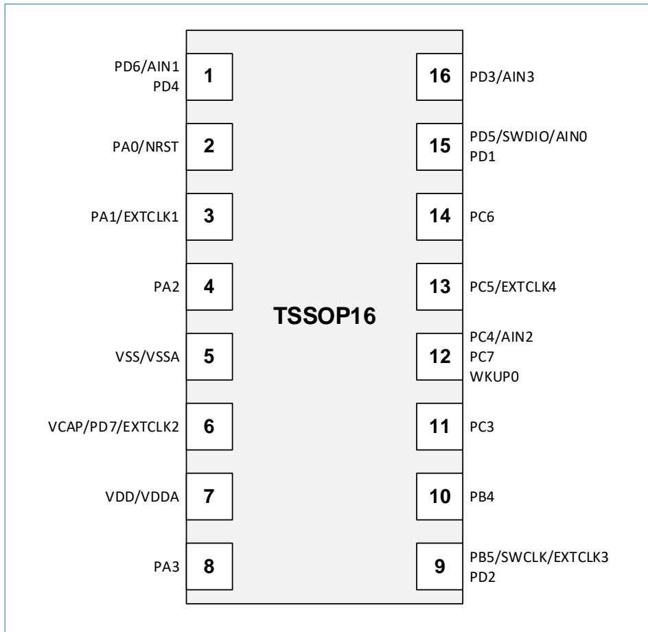
图 6-3 TSSOP16 封装
