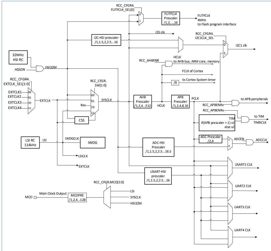
图 3-4 时钟树
