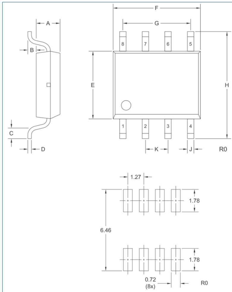
图 7-6 SOP8 封装尺寸
