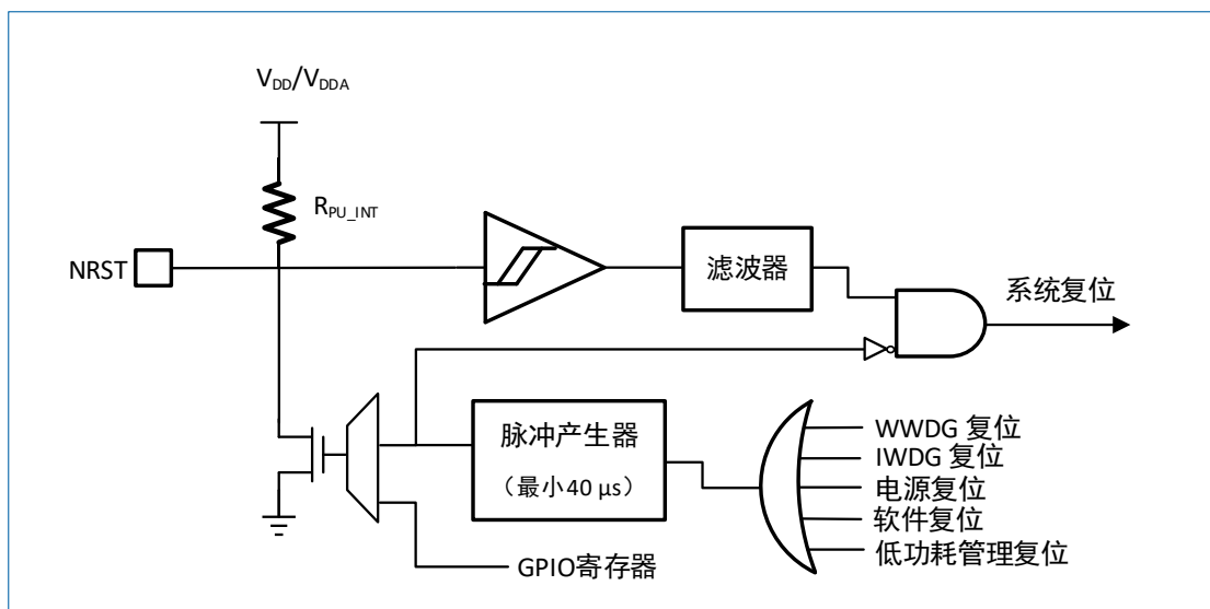
图 3-3 复位电路
