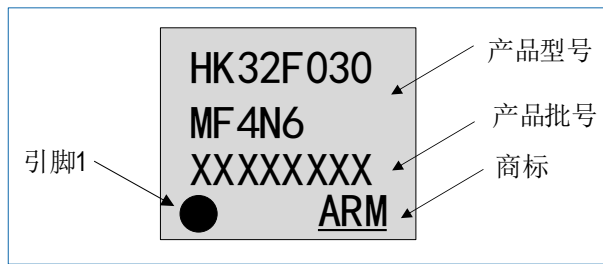
图 7-7 QFN20 HK32F030MF4N6 丝印示例
