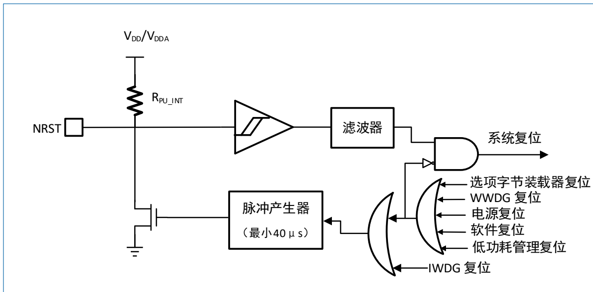
图 6-1 复位电路
