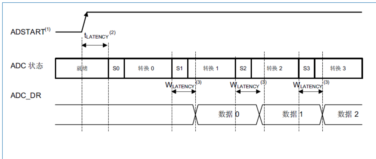
图 11-5 模数转换时序
