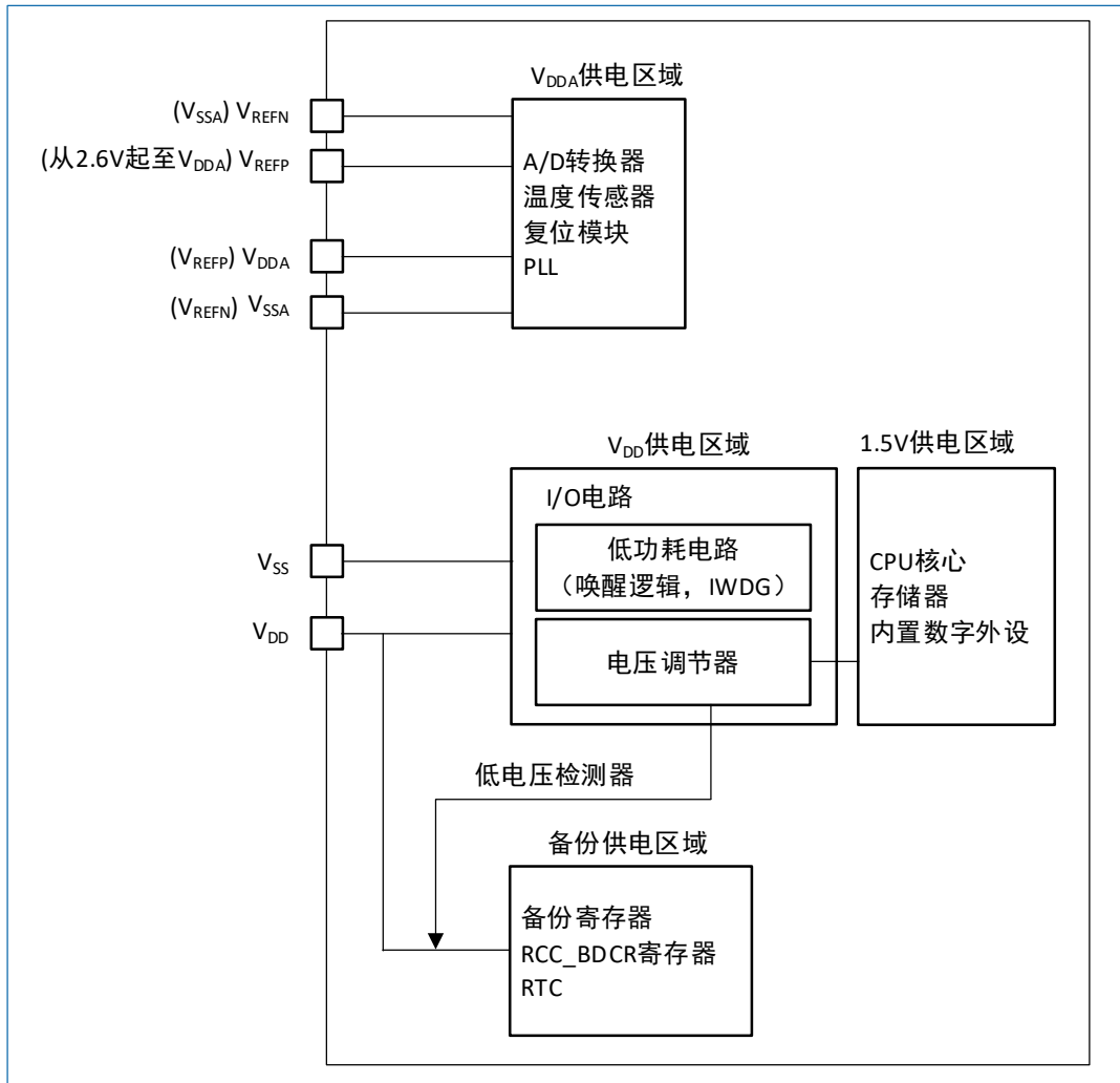
图 5-1 电源框图
