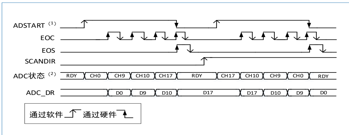
图 11-7 单次序列转换, 软件触发
