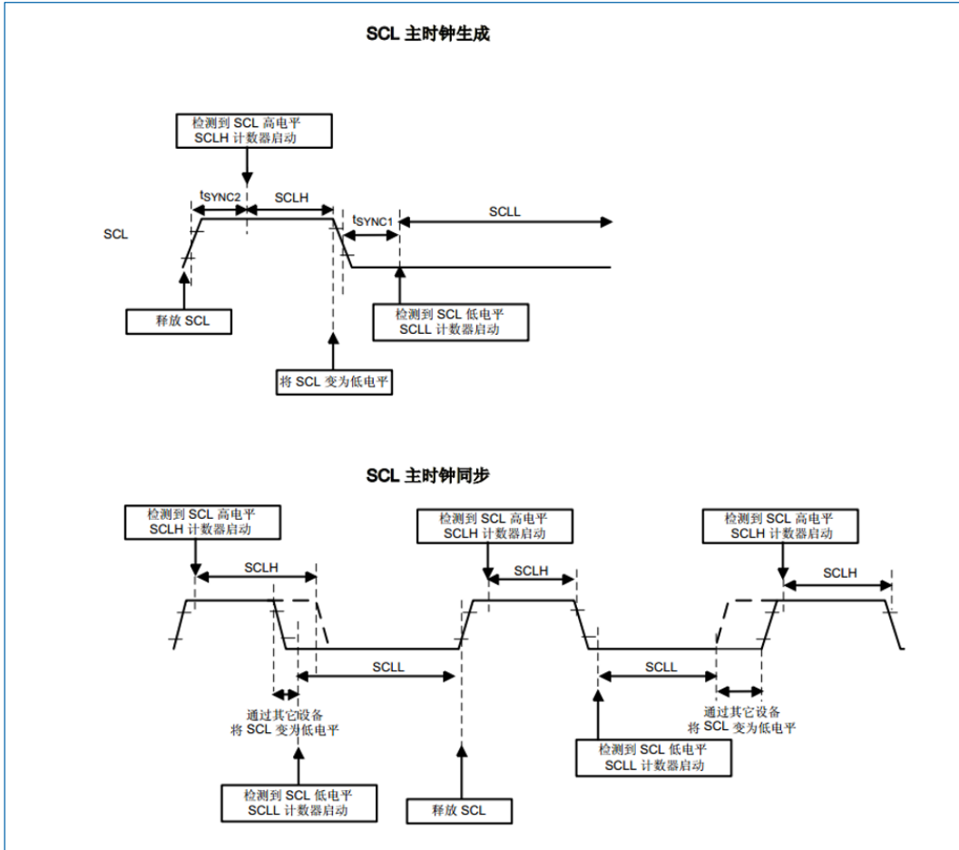
图 22-14 主时钟生成
