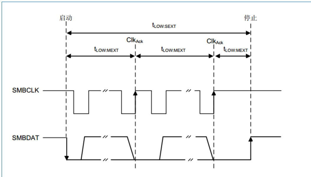
图 22-24 t_{\text{LOW:SEXT}} 和 t_{\text{LOW:MEXT}} 的超时间隔
