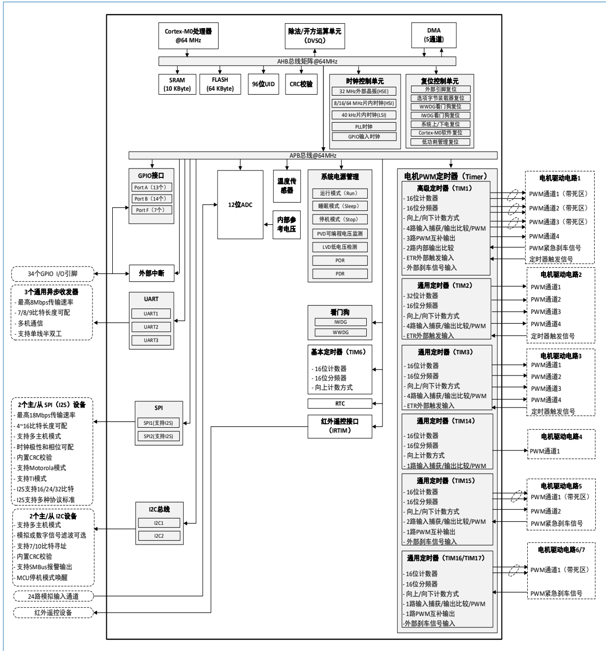
图 2-1 HK32C105S8T7 功能框图
