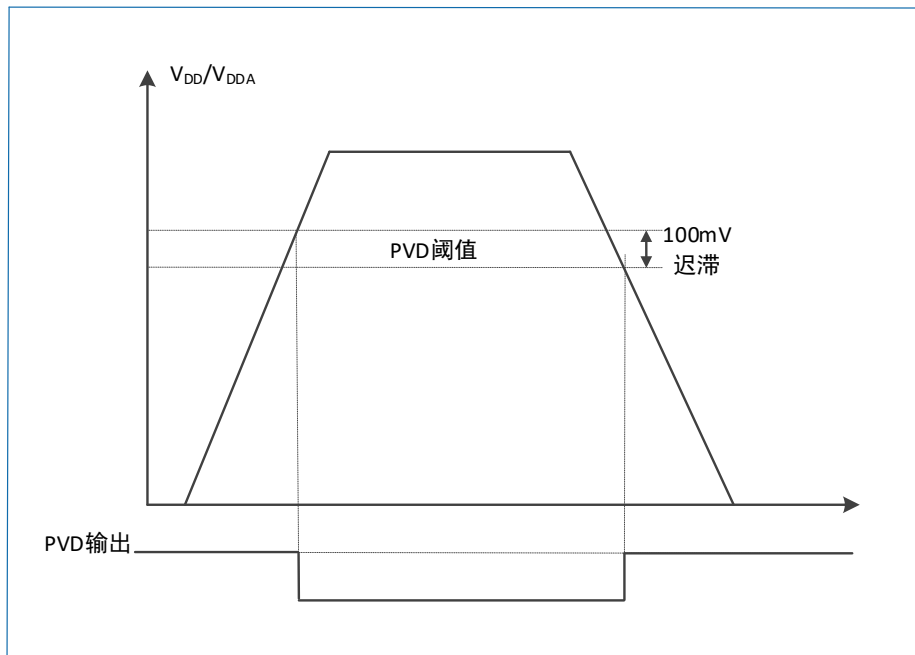
图 5-3 PVD 的门限
