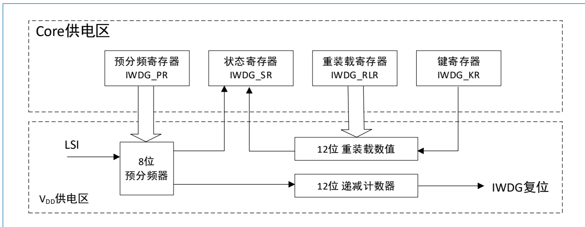
图 20-1 IWDG 框图
