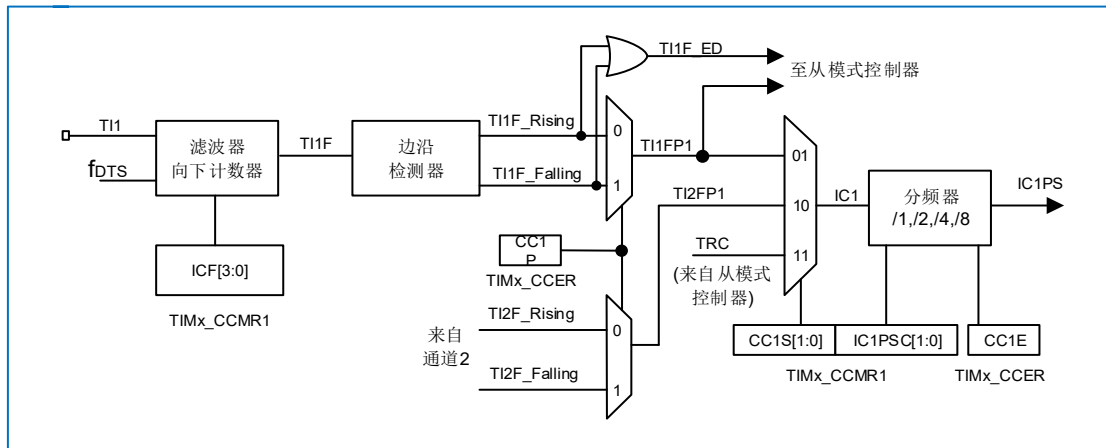
图 14-27 捕获/比较通道（如：通道 1 输入部分）
