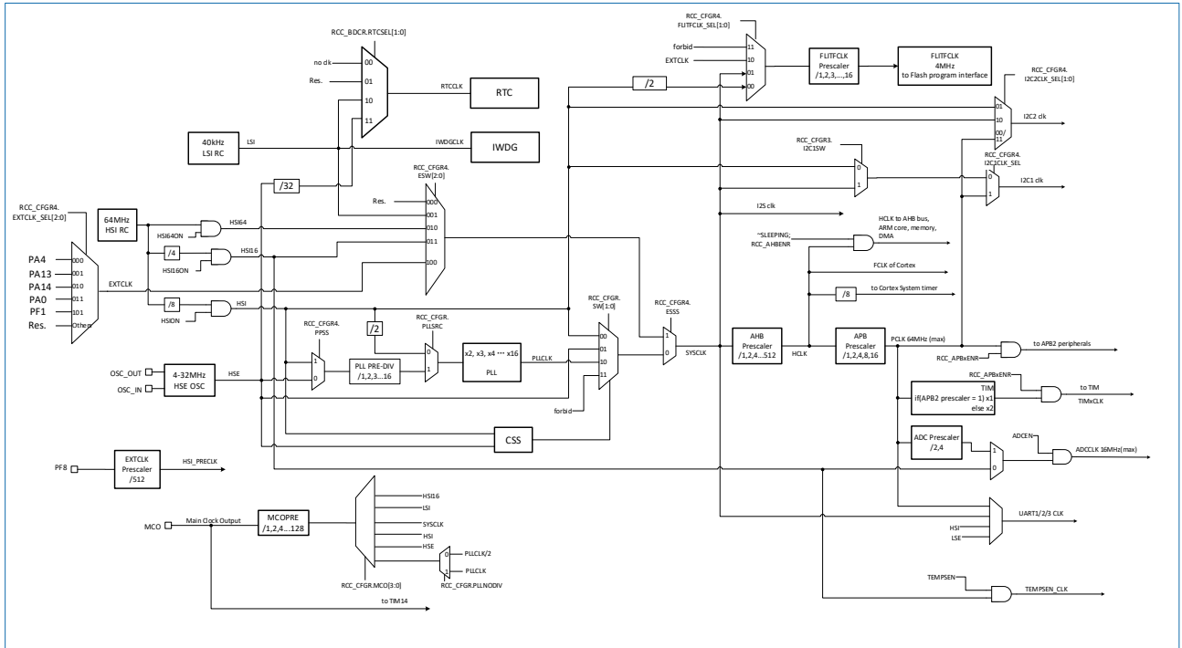
图 6-2 时钟树
