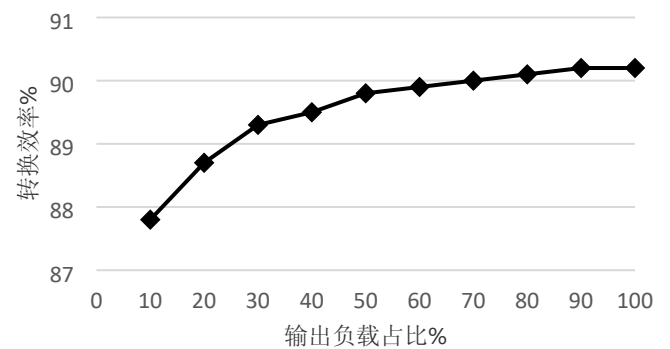
负载效率曲线
