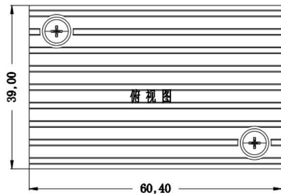
标准型+散热器 60.4*39*27.7mm
