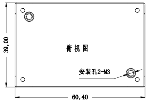
标准型 60.4*39*12.7mm
