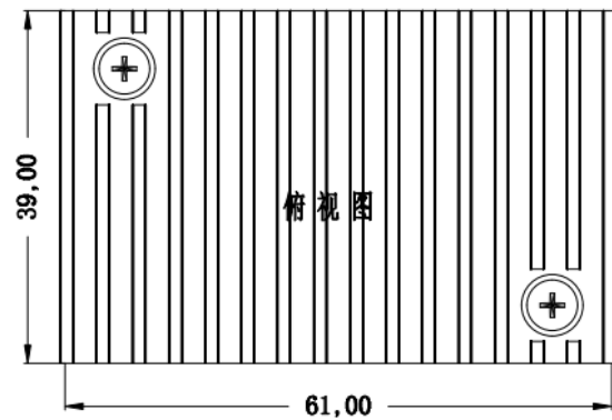
标准型+散热器 61.0*39.0*27.7mm
