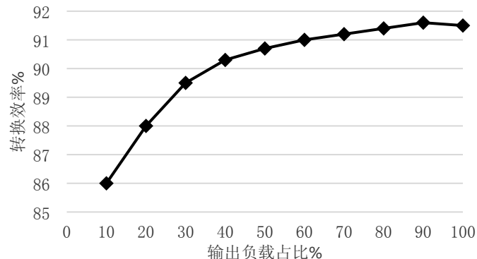
负载效率曲线
