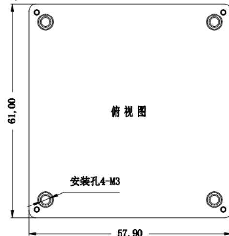
标准型 61*57.9*12.7mm
