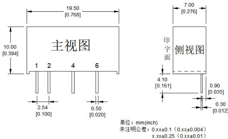
封装尺寸图
