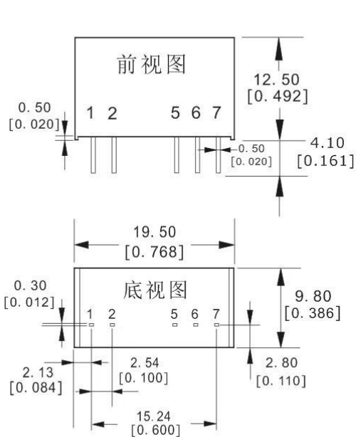
封装尺寸图
